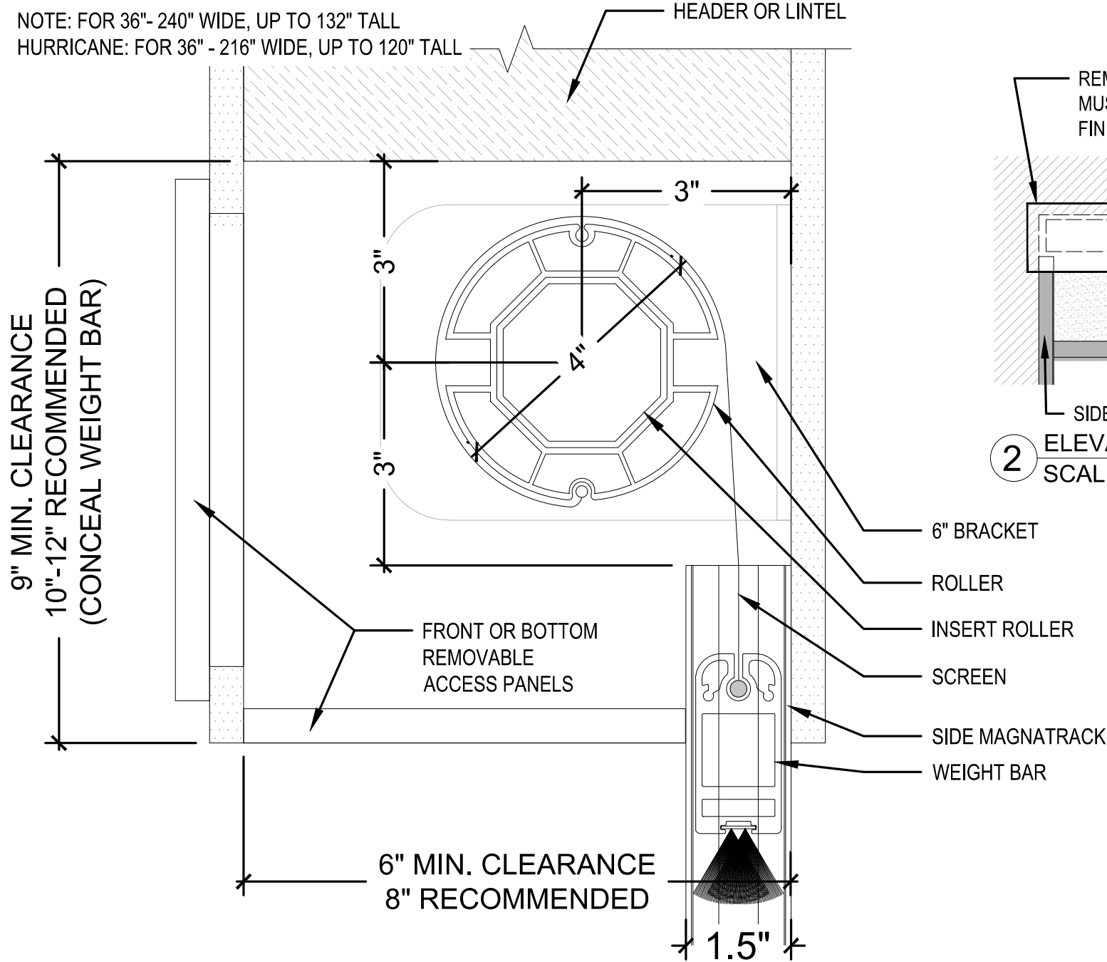
1 SECTION SCALE: 6" = 1'-0"
